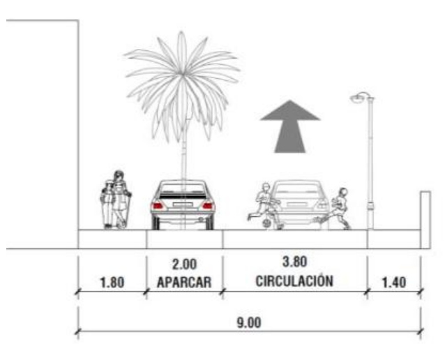
Ilustración 37. Sección Calle de Convivencia de 9 metros.
